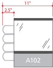
INFO2EVWIN-4L 10-11/16"h x 8-1/2"w (OD) 7"h x 8-1/2"w Display Insert 7-5/8"h x 8-1/2"w Window (OD) 3" ADA Insert
