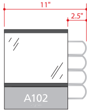
INFO2EVWIN-4R 10-11/16"h x 8-1/2"w (OD) 7"h x 8-1/2"w Display Insert 7-5/8"h x 8-1/2"w Window (OD) 3" ADA Insert
