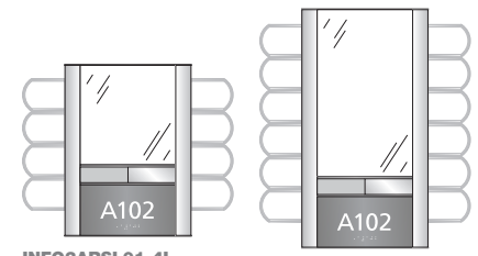
INFO2ARSL01-4L 10.08"h x 7.5"w (OD) 5.838"h x 6"w - Display Area 1.16"h - Slider 3"h - ADA Band
