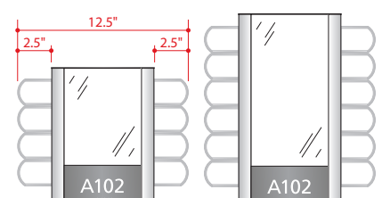
INFO2AR01-4RL 10.08"h x 7.5"w (OD) 7"h x 6"w - Display Area 3"h - ADA Band
