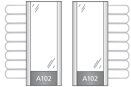
INFOAR01-8L 17.83"h x 7.5"w (OD) 14.75"h x 6"w - Display Area 3"h - ADA Band
