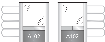
INFOARSL01-4L 10.08"h x 7.5"w (OD) 5.838"h x 6"w - Display Area 1.16"h - Slider 3"h - ADA Band
