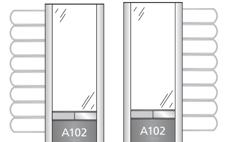
INFOARSL01-8L 17.83"h x 7.5"w (OD) 13.588"h x 6"w - Display Area 1.16"h - Slider 3"h - ADA Band
