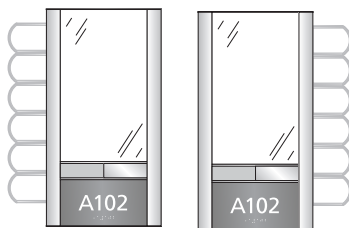
INFO2ARSL01-6L 14.08"h x 7.5"w (OD) 9.838"h x 6"w - Display Area 1.16"h - Slider 3"h - ADA Band
