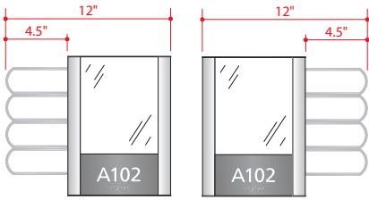
INFOAR01-4L 10.08"h x 7.5"w (OD) 7"h x 6"w - Display Area 3"h - ADA Band
